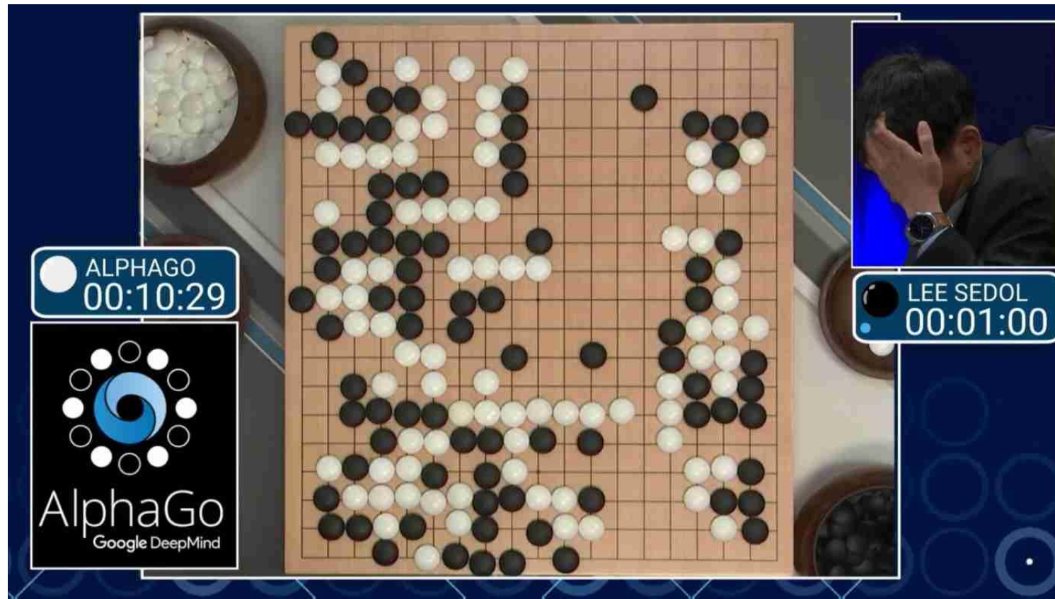
Hình 6: AlphaGo
